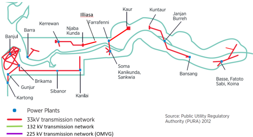
冈比亚电网现状图
